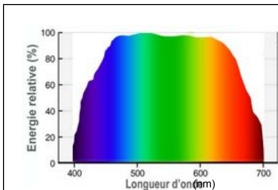
Figure 8 : spectre électromagnétique d'une diode électroluminescente cms n°1
