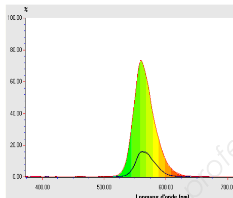
Figure 9 : spectre électromagnétique d'une diode électroluminescente cms n°2
