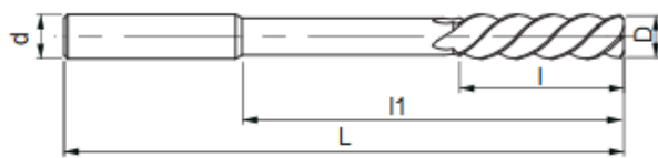
Alésoir machine spécial coupe al et mg hélice à gauche pour alésage débouchant
