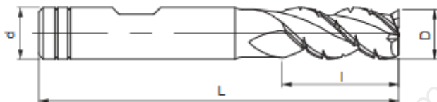
Fraises à profil brise copeau
