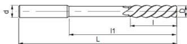
Alésoir machine spécial coupe al et mg hélice à gauche pour alésage débouchant
